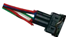
0250.996.037 - Chicote 5 vias 4 fios reparo adaptação bomba combustível Ford KA/Fiesta/Courier
