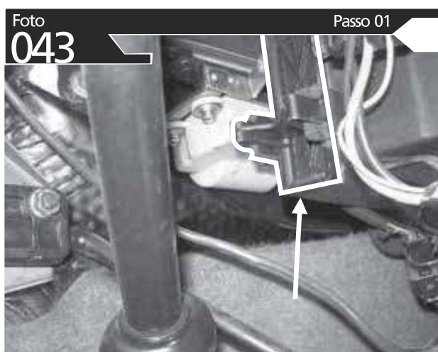
O FILTRO ESTÁ LOCALIZADO AO LADO E ACIMA DO PEDAL DO ACELERADOR
