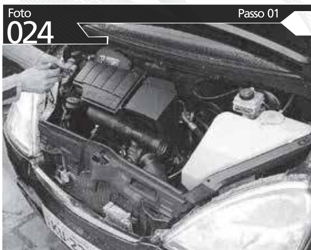
O FILTRO DE CABINE ESTÁ LOCALIZADO AO CENTRO SOB O CAPÔ. RETIRE OS PARAFUSOS INDICADOS, FECH E O CAPÔ E RETIRE A CARENAGEM DE PROTEÇÃO
